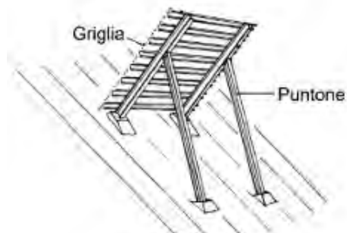
Figura 4.1 - Schematizzazione di un ponte da neve (adattata da Margreth, 2007).
